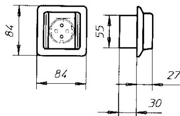
Måttritning
